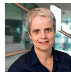
N. Waddel
